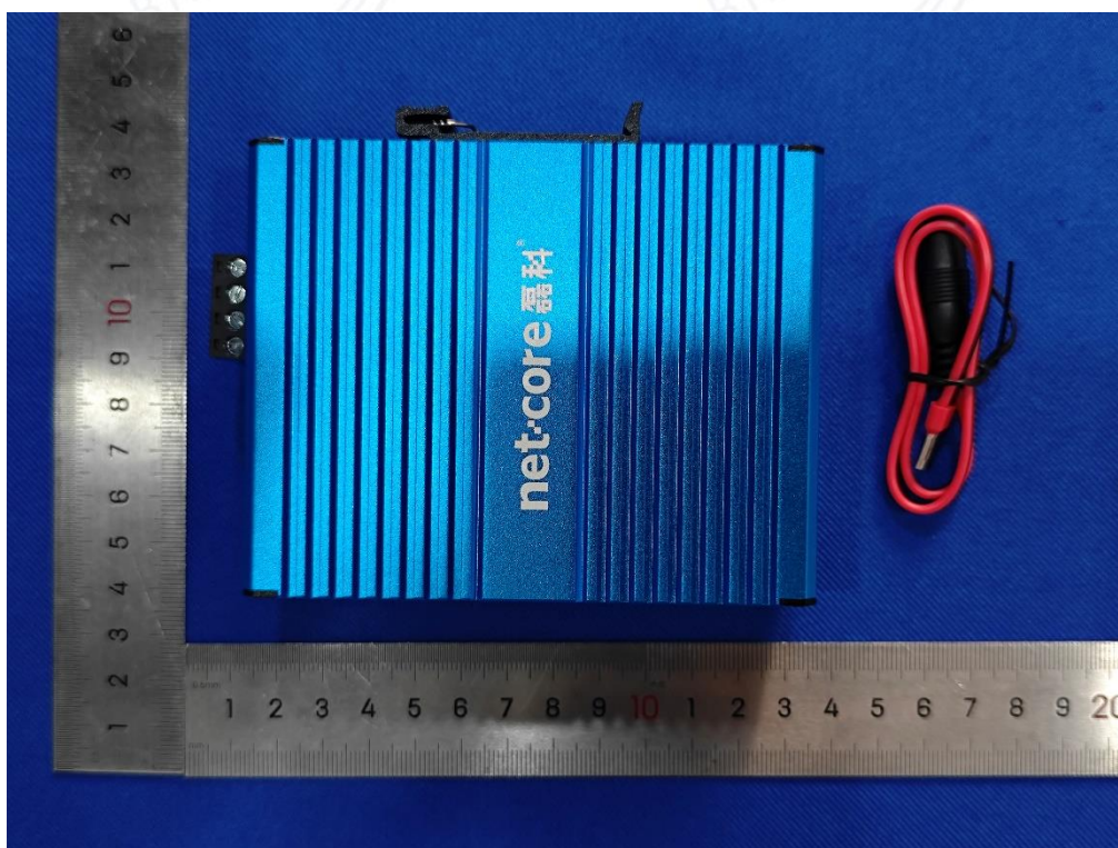
照片 1 产品外观
